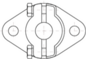
Anschlagflansch 32
